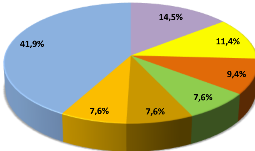
TYCHY
